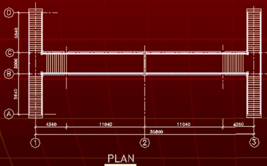
Puentes Prefabricados
