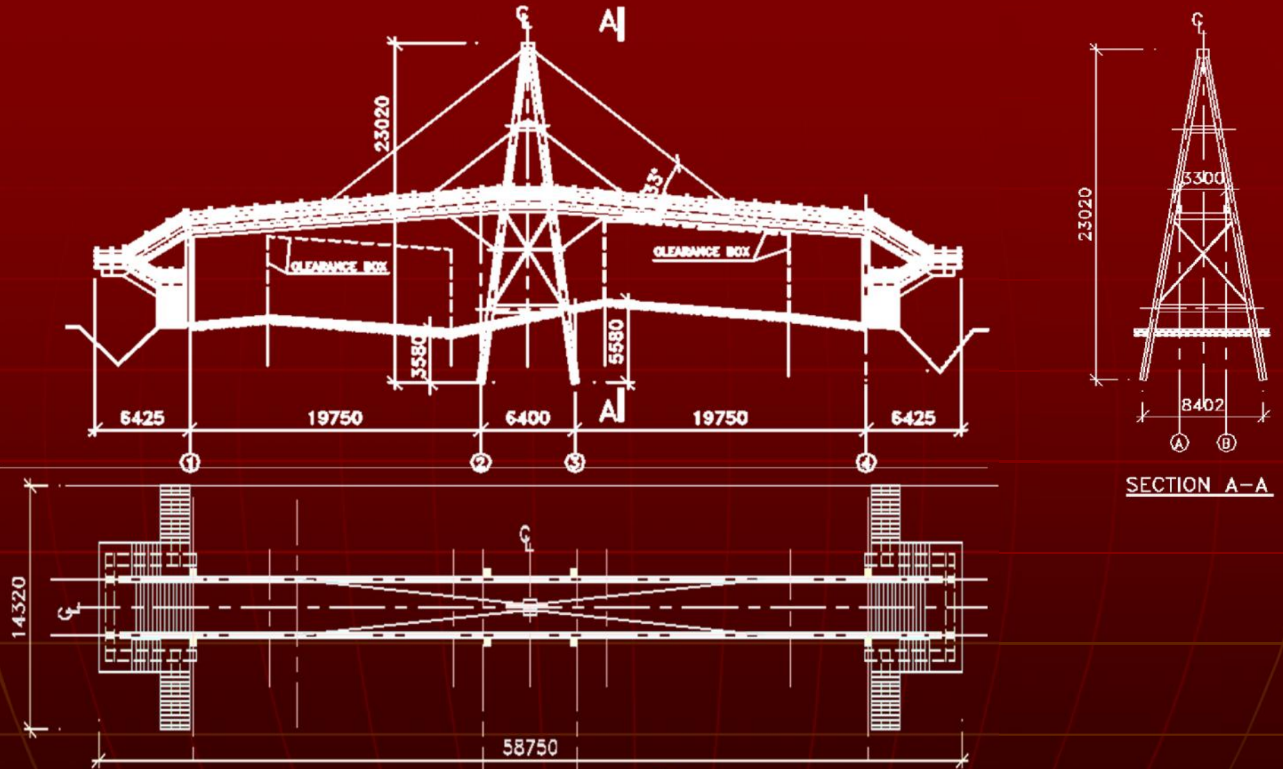
Esquema General Puente Peatonal, Zip Buena Vista
